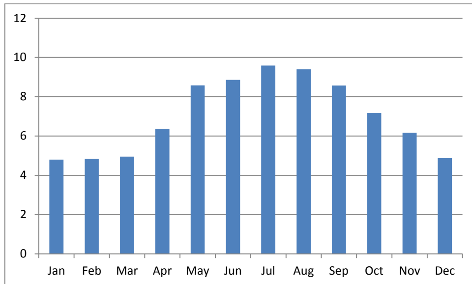
Figure 3 : Vitesse moyenne à 50m d'altitude
