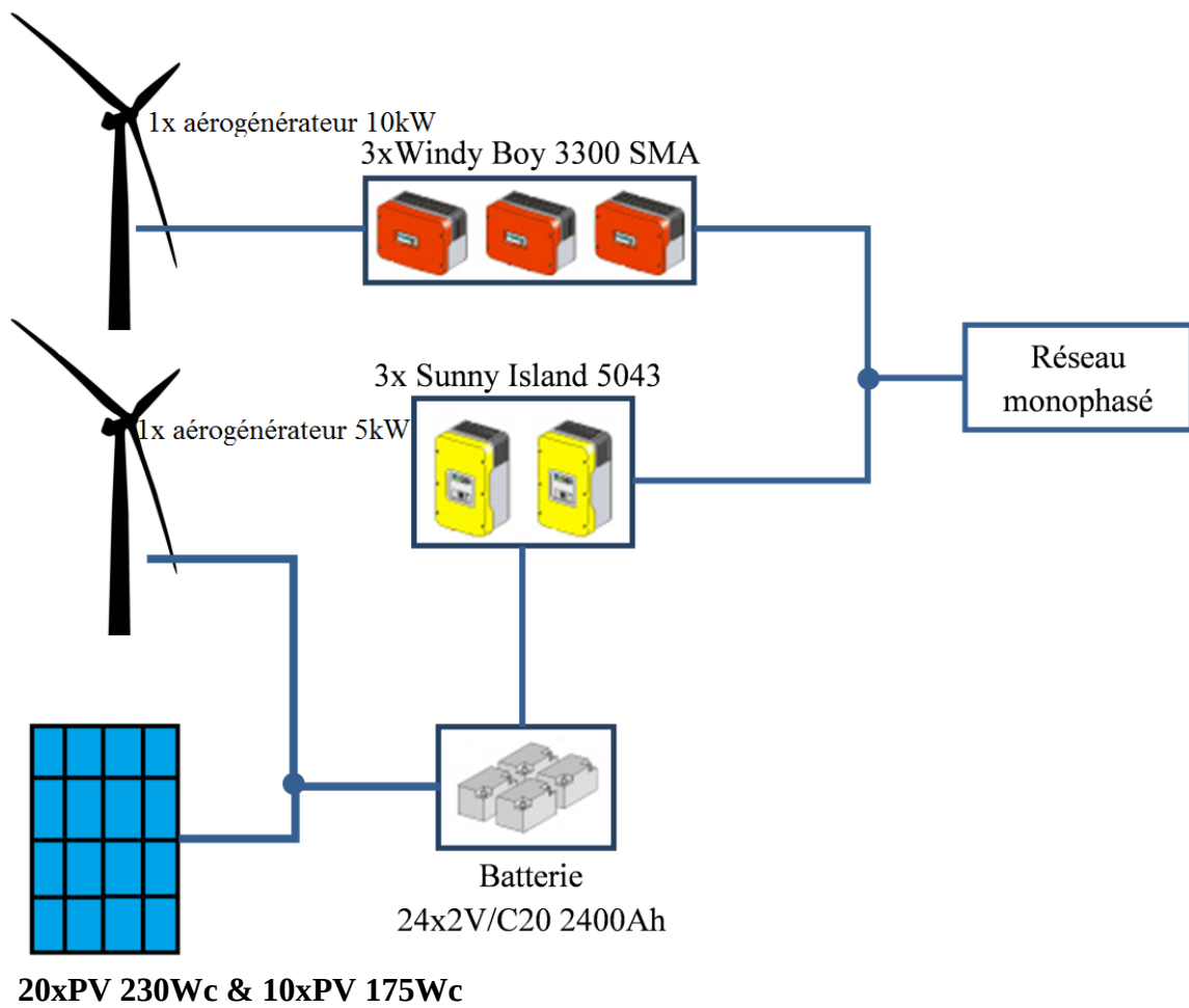
Figure 12 : Schéma synoptique de la centrale hybride isolé d'Ifovona
