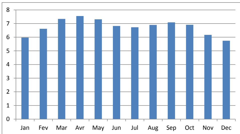
Figure 1: Courbe d'irradiation solaire en kWh/m²/j du village d'Ambolobozobe
