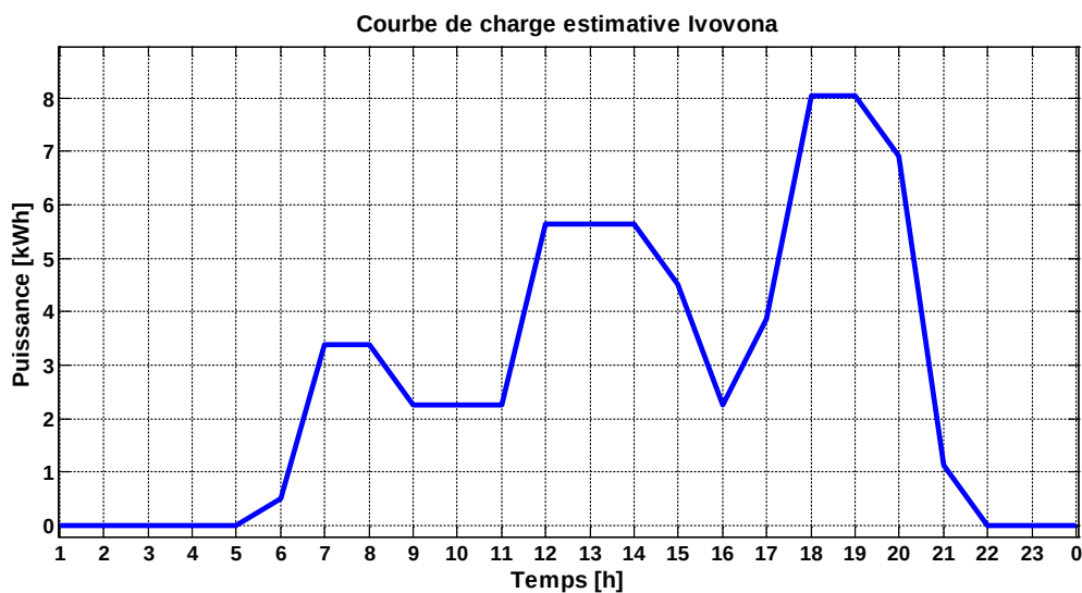
Figure 9: Courbe des charges estimative de la consommation d'énergie du village d'Iovona
