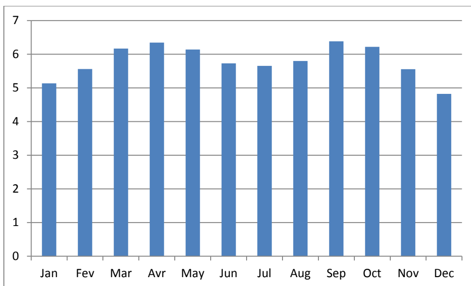
Figure 2: Courbe d'irradiation solaire en kWh/m²/j du village d'Ivovona
